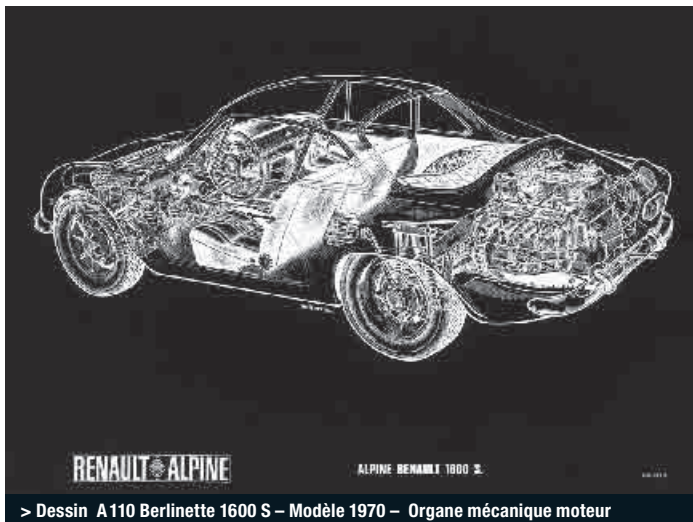
> Dessin A 110 Berlinette 1600 S – Modèle 1970 – Organe mécanique moteur
