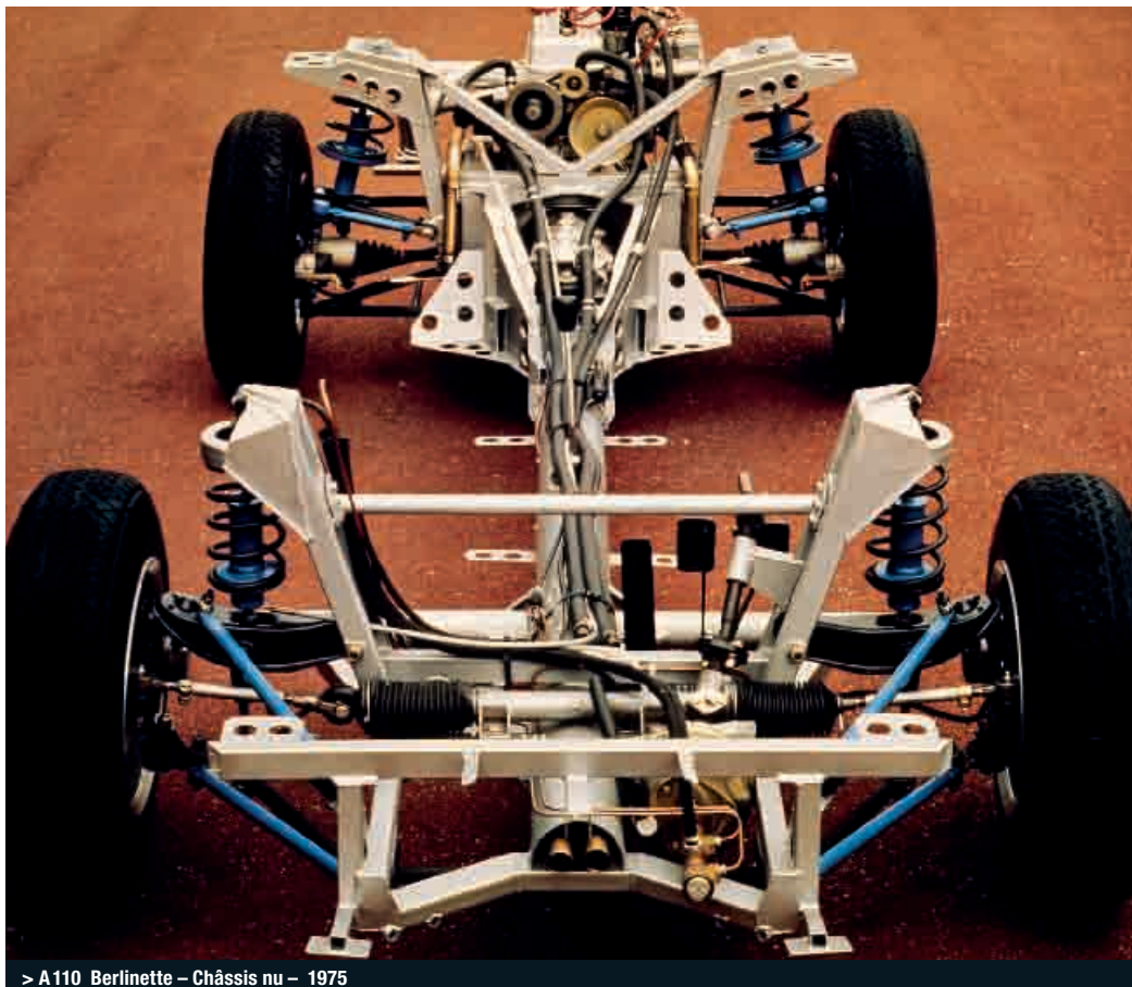
> A 110 Berlinette – Châssis nu – 1975
